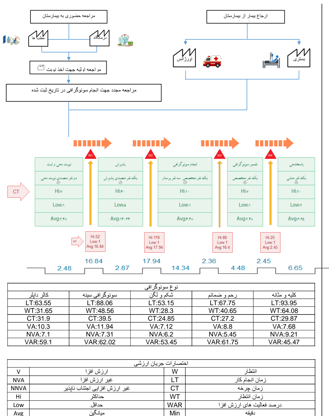
شکل ۱: نقشه اولیه جریان ارزش فرآیند سونوگرافی
